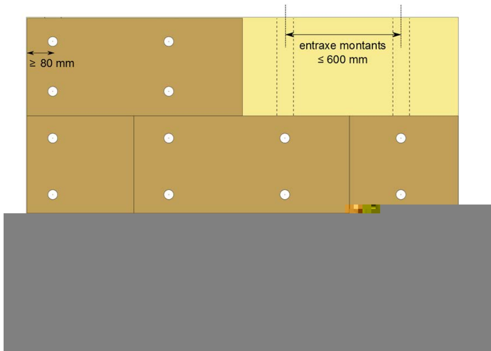
4 vis à rosace par panneau (2 vis par montant)
