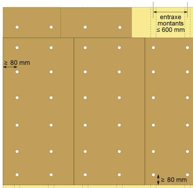
12 vis à rosace par panneau (6 vis par montant)
