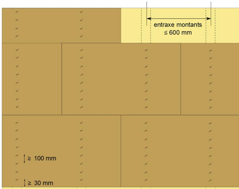
16 agrafes par panneau (8 agrafes par montant)
