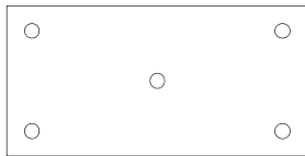
Figure 1a : Plans de chevillage - panneaux de dimensions 1000 × 500 mm
