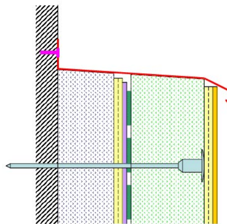
Figure 2d : nouvelle couverture inversée avec dépose de l'ancienne
