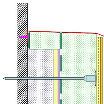
Figure 2f : nouvelle couverture avec dépose de l'ancienne, disquage de l'ancienne ITE et collage d'un nouvel isolant
